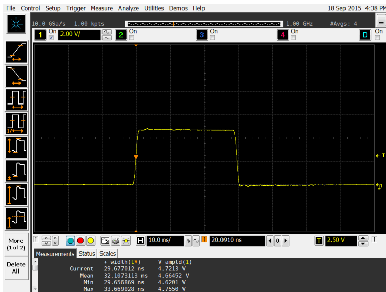
Рис. 3. Рекомендуемая форма внешнего импульса запуска.
