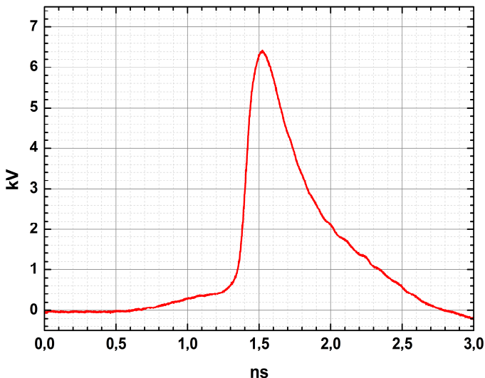
Рис.2. Типичная форма выходного импульса генератора PPM0731 на согласованной нагрузке с импедансом 50 Ом.
